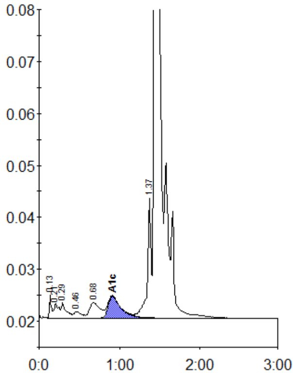
Peak table - ID: 11947786
