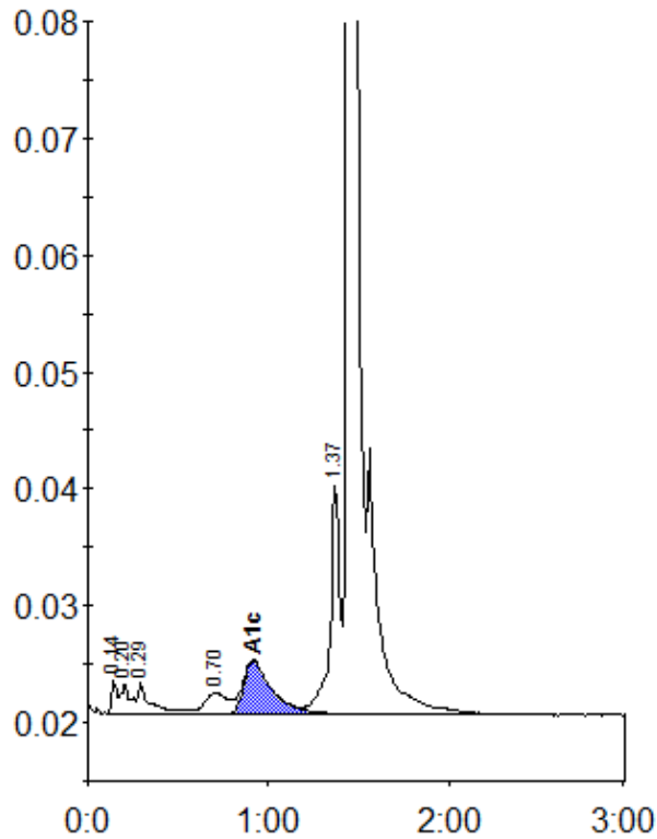
Peak table - ID: 11965608
