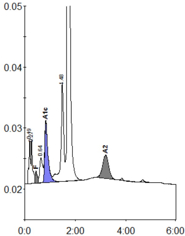
Peak table - ID: 11797112
