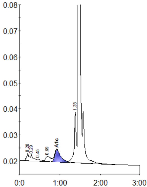
Peak table - ID: 11853854
