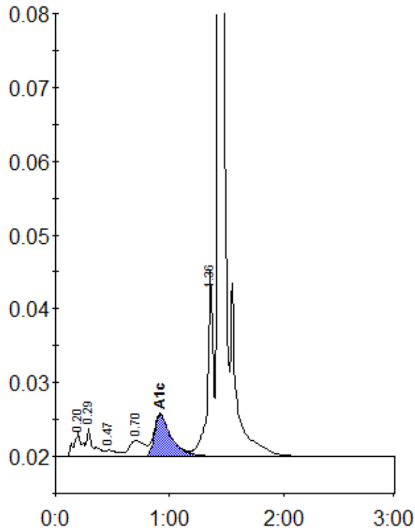
Peak table - ID: 11795657
