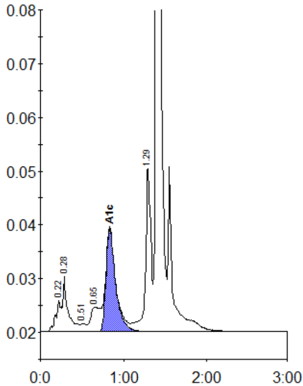
Peak table - ID: 11483209
