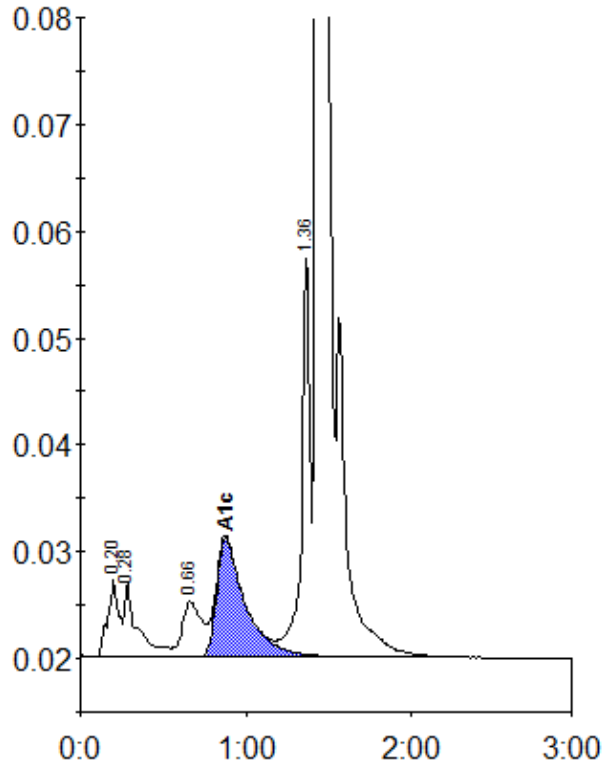
Peak table - ID: 11797547
