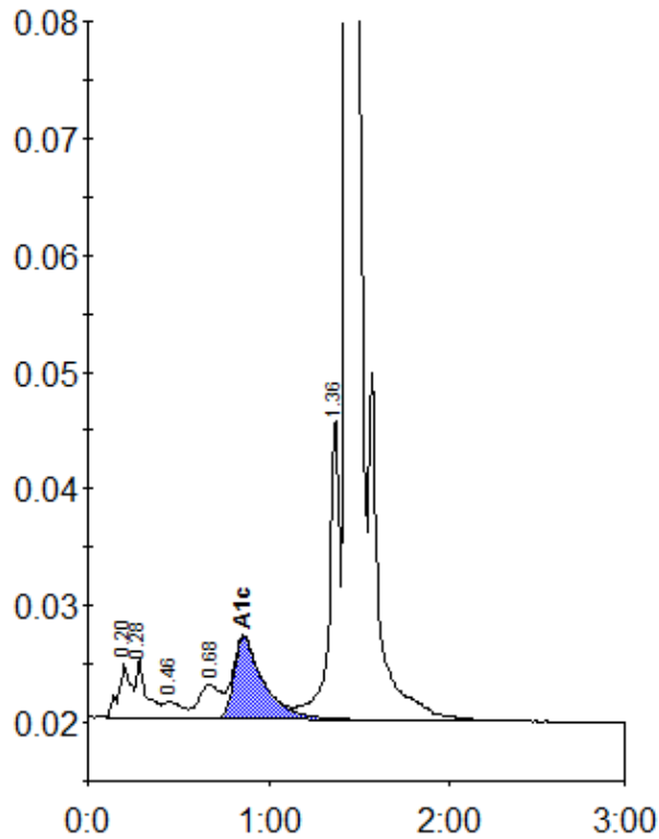
Peak table - ID: 11795726
