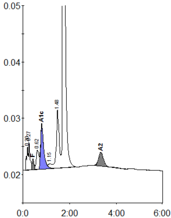
Peak table - ID: 11667483
