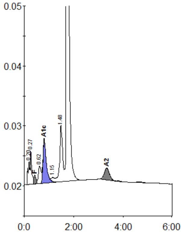
Peak table - ID: 11638538
