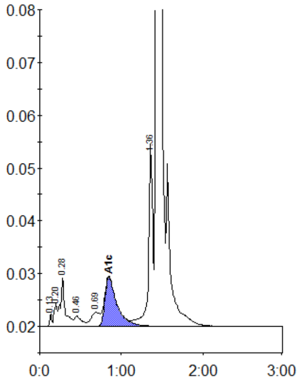
Peak table - ID: 11485217
