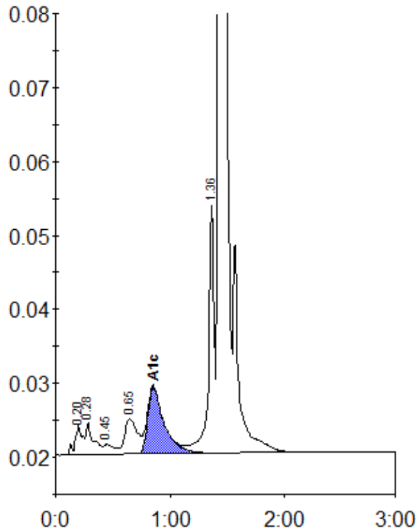
Peak table - ID: 11646804
