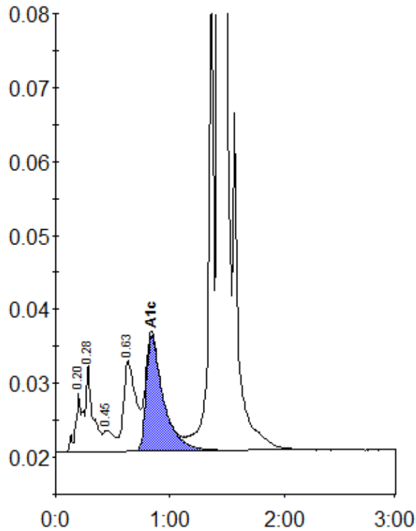
Peak table - ID: 11477425
