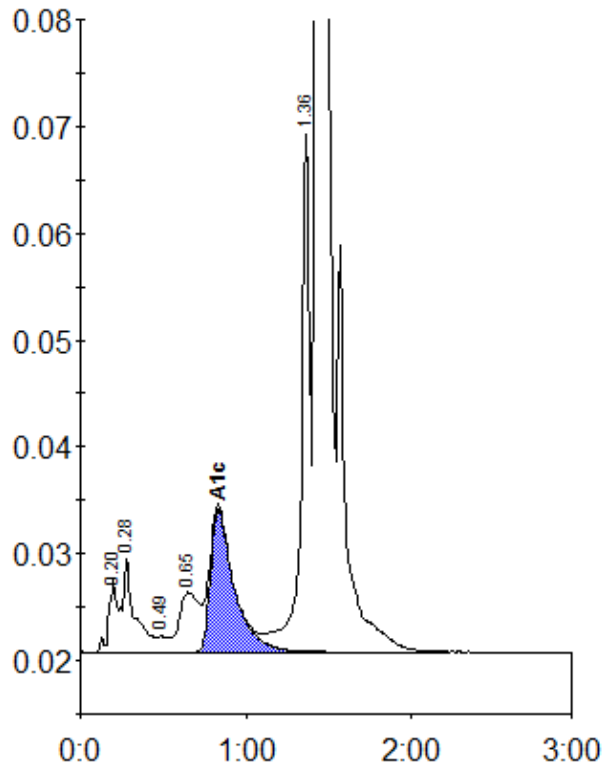
Peak table - ID: 11646537
