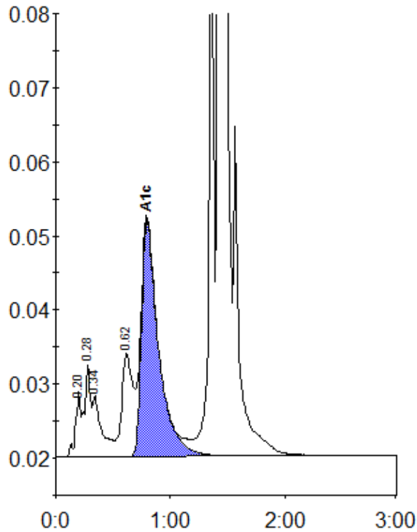
Peak table - ID: 11483471
