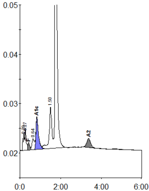
Peak table - ID: 11463974
