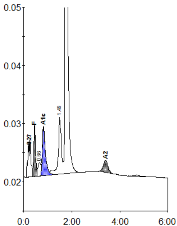
Peak table - ID: 11491761
