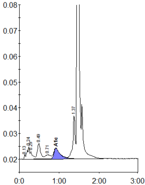
Peak table - ID: 11486134
