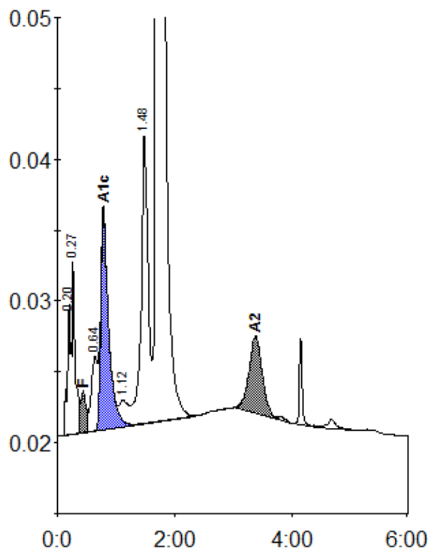
Peak table - ID: 11487743
