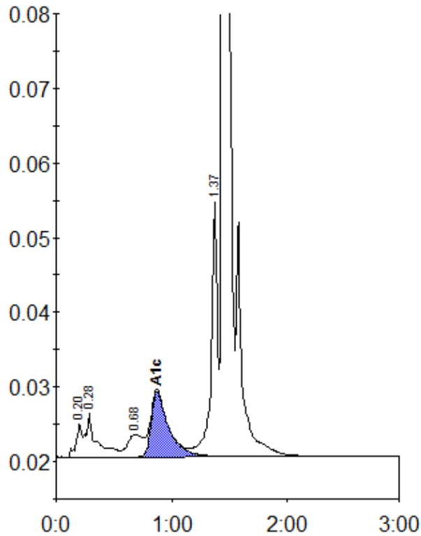
Peak table - ID: 11479159
