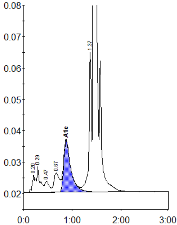
Peak table - ID: 11485824
