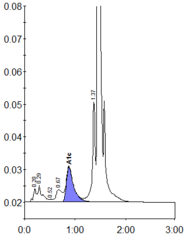
Peak table - ID: 11486484
