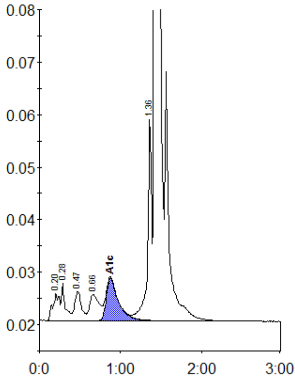
Peak table - ID: 11479527
