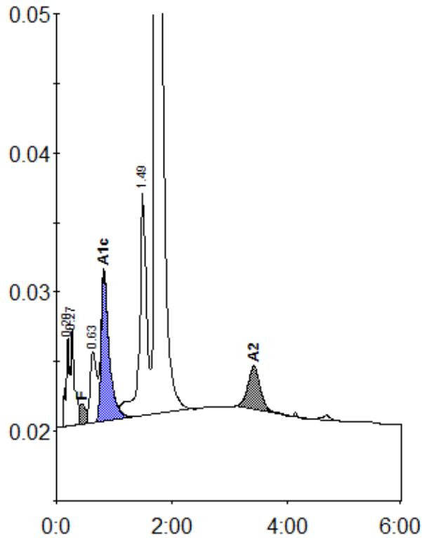
Peak table - ID: 100019793
