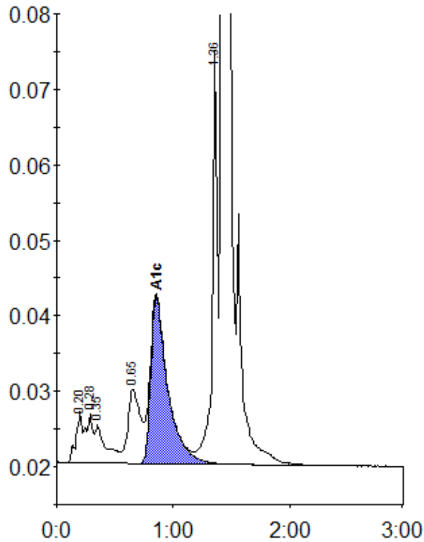
Peak table - ID: 11494755
