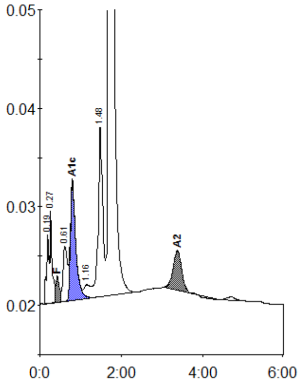
Peak table - ID: 11493958
