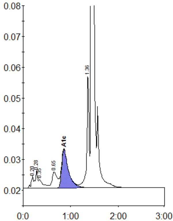
Peak table - ID: 11512918
