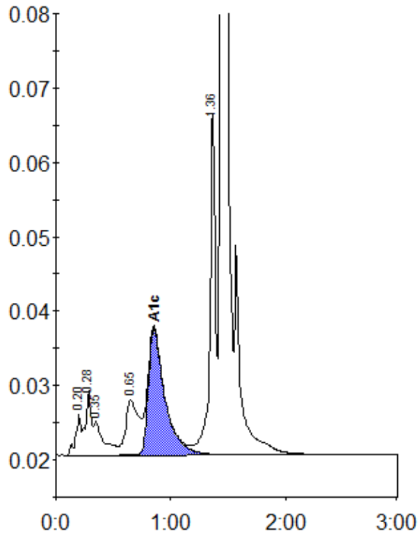
Peak table - ID: 11447293
