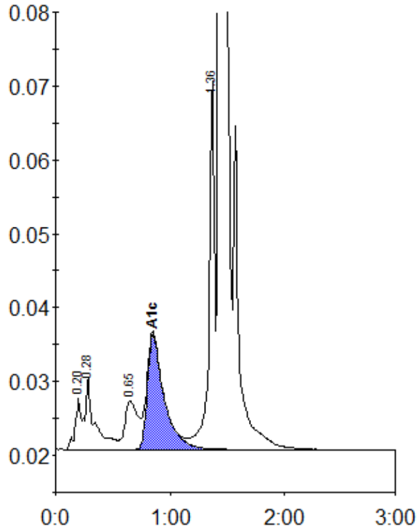
Peak table - ID: 11631169
