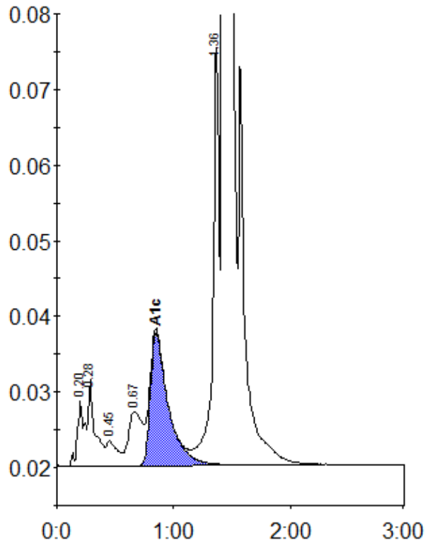
Peak table - ID: 11492481
