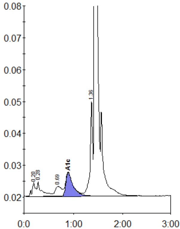
Peak table - ID: 11460341
