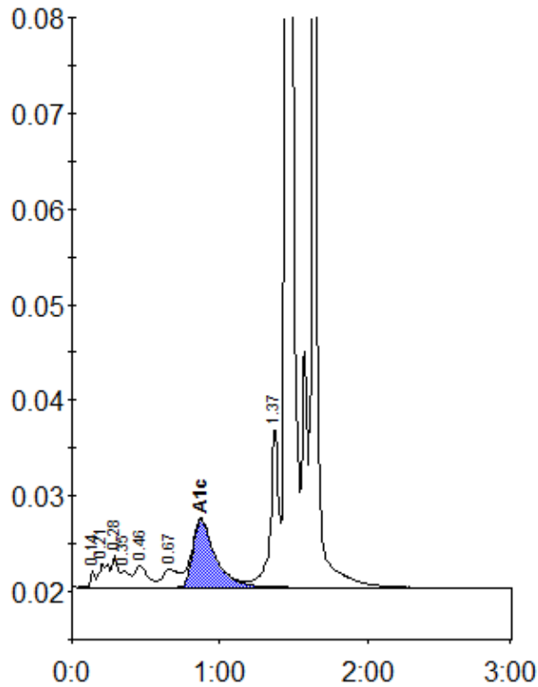
Peak table - ID: 11466169
