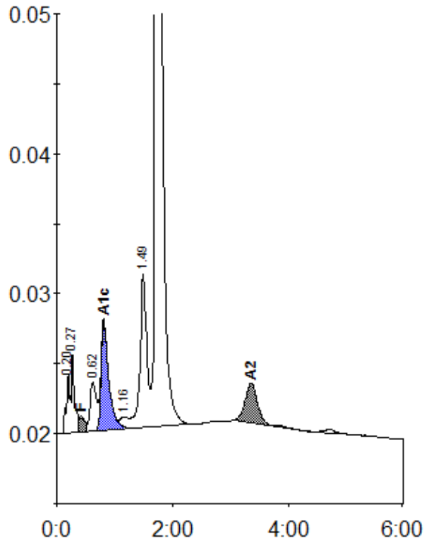
Peak table - ID: 11358944
