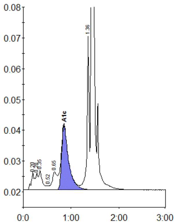
Peak table - ID: 11455190
