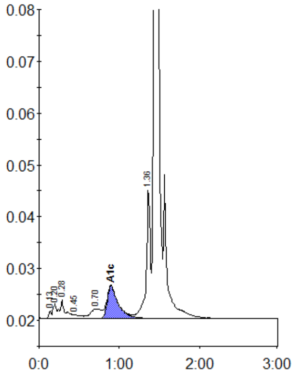
Peak table - ID: 11466444
