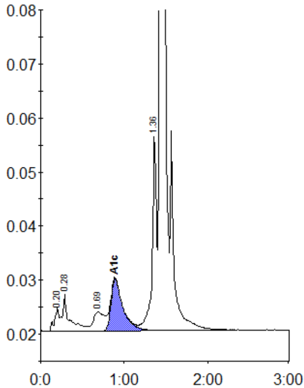
Peak table - ID: 11470784
