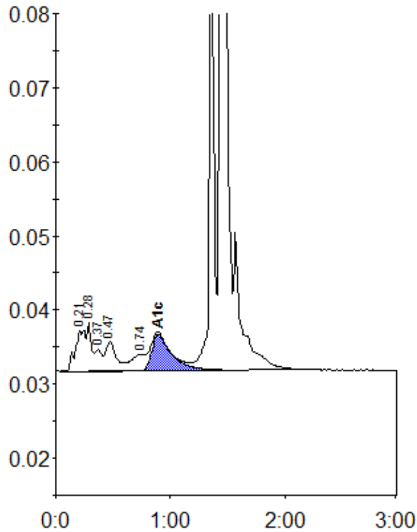
Peak table - ID: 10997581
