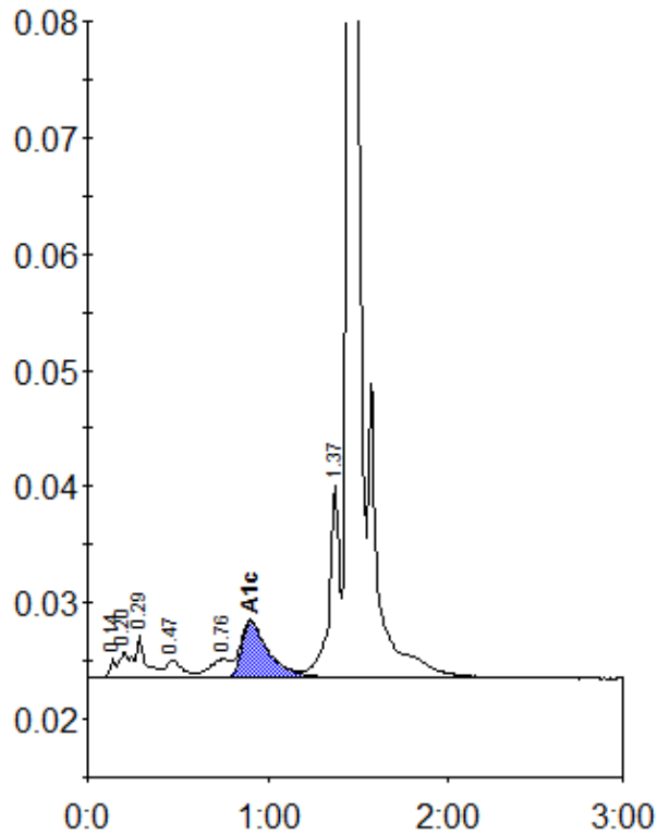
Peak table - ID: 11187194
