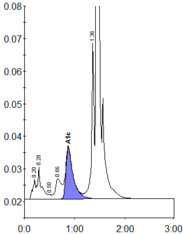
Peak table - ID: 11451791
