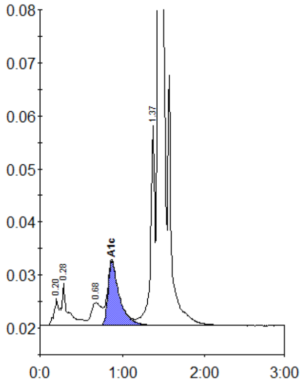
Peak table - ID: 11422319
