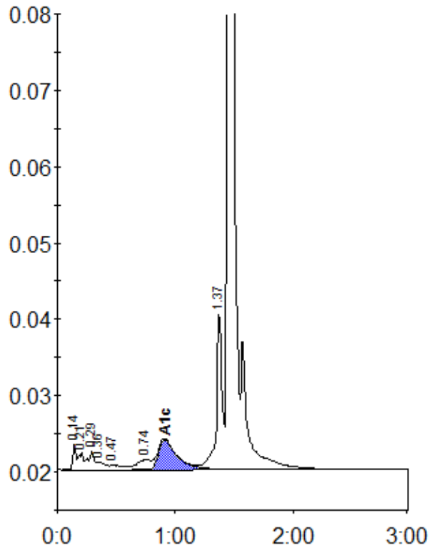
Peak table - ID: 11414280
