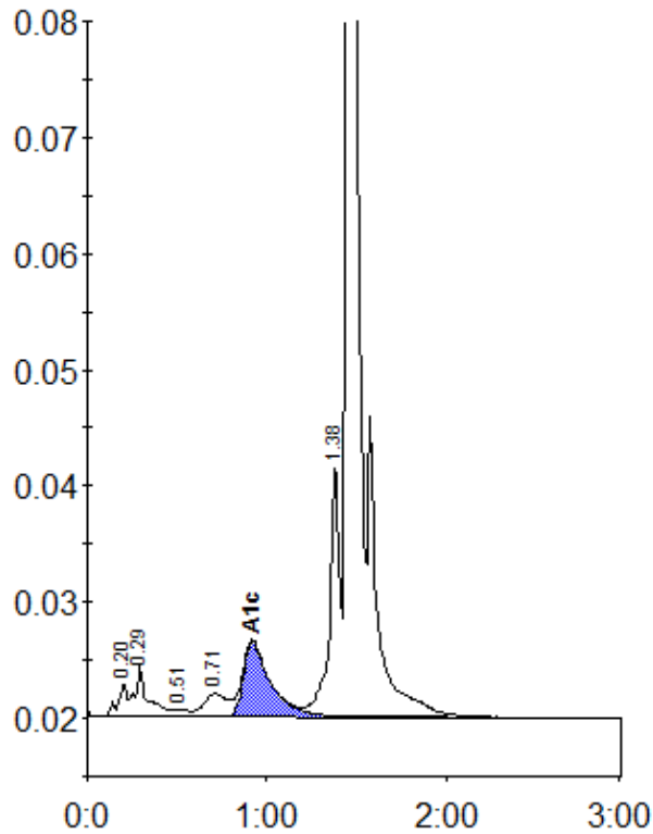
Peak table - ID: 11187669
