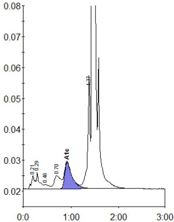
Peak table - ID: 11414488
