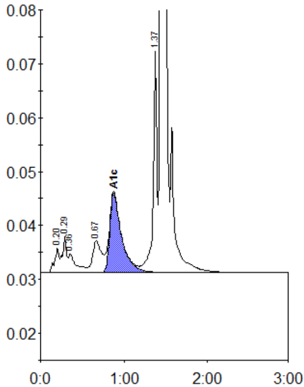
Peak table - ID: 11414796
