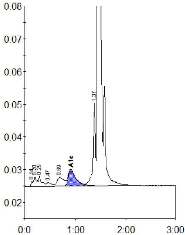
Peak table - ID: 11414912
