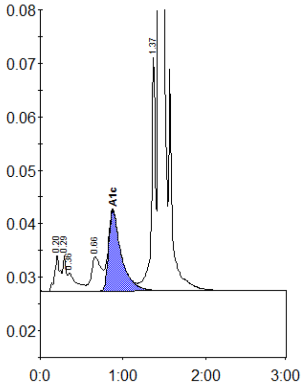
Peak table - ID: 11298382
