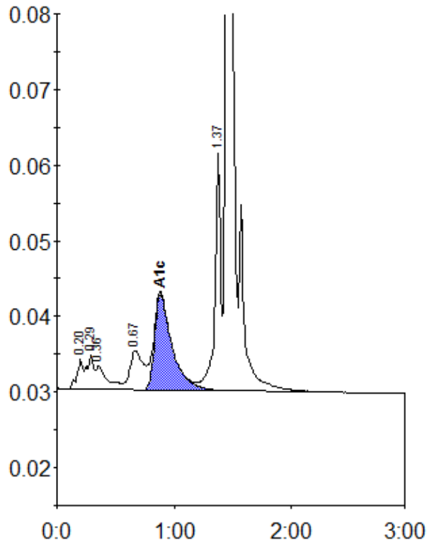
Peak table - ID: 11414961
