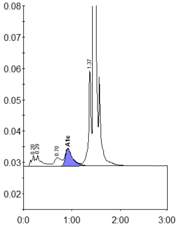
Peak table - ID: 11414975
