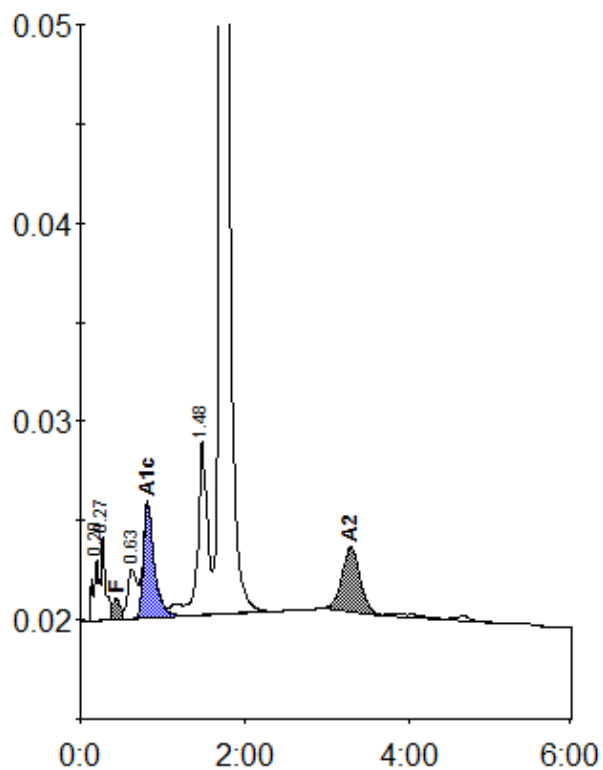
Peak table - ID: 008635521
