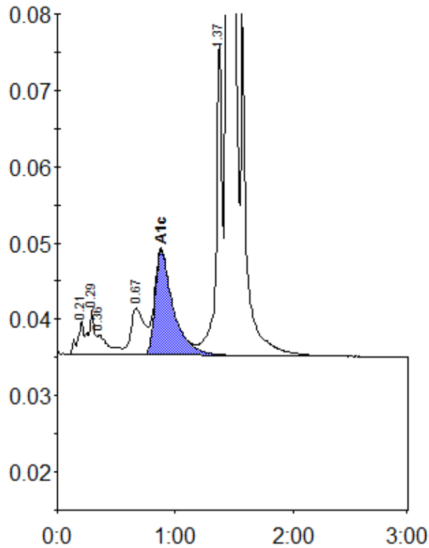
Peak table - ID: 11182686
